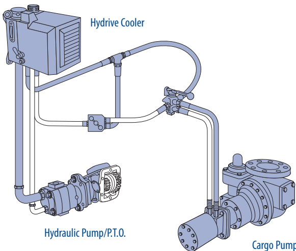
TLGLF4 cutaway
