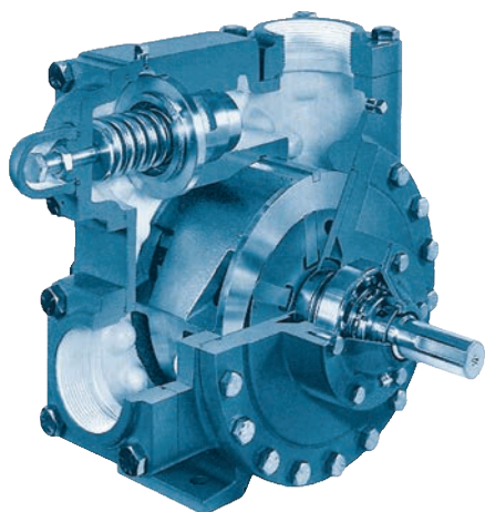
LGLD4 (разрез)
