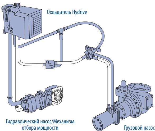
TLGLF4 (разрез)
