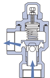
РИС. 5. Работа перепускного клапана
