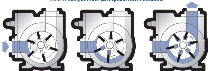
РИС. 1. Как работает шиберный насос Blackmer
