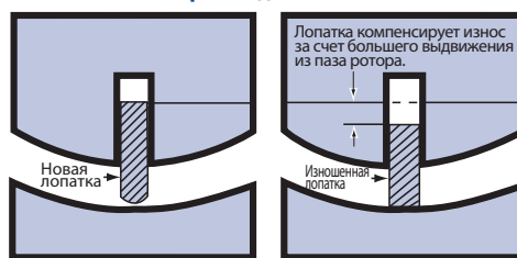
РИС. 2. Как шиберные лопатки Blackmer поддерживают производительность
