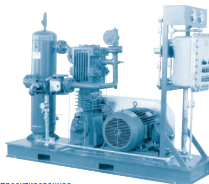
Специально спроектированная компрессорная установка для перекачки сжиженного нефтяного газа
