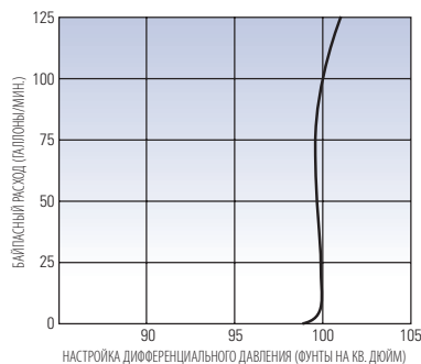
РИС. 4. Кривая зависимости байпасного объема и давления BV1 1/2
