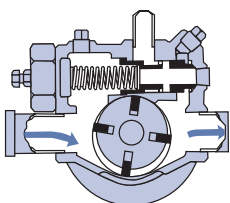
РИС 3. Комбинированный предохранительный/перепускной клапан
