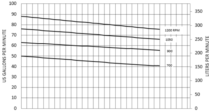
1 cP (30 SSU)
