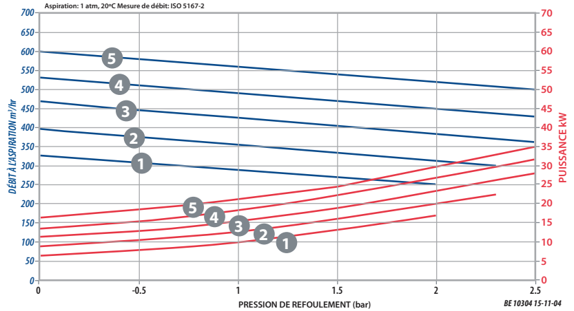
Débit (m 3 /h) / Puissance (kW)
