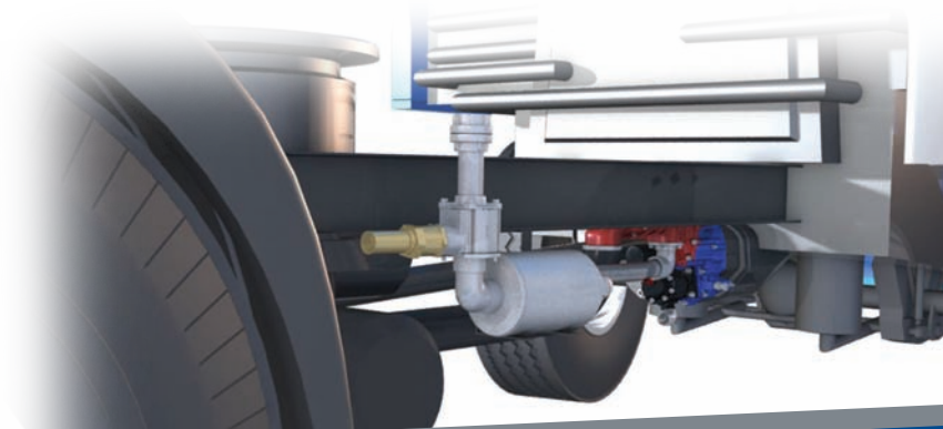
Limiteur de couple intégré dans le module PTO
