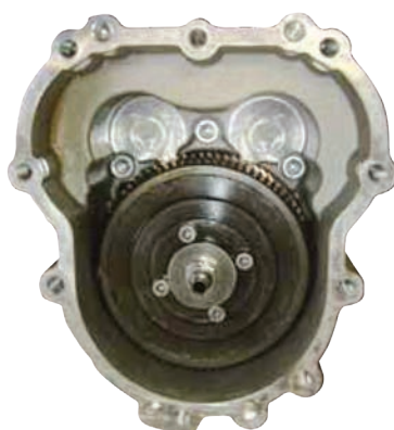
Limiteur de couple intégré dans le module PTO
