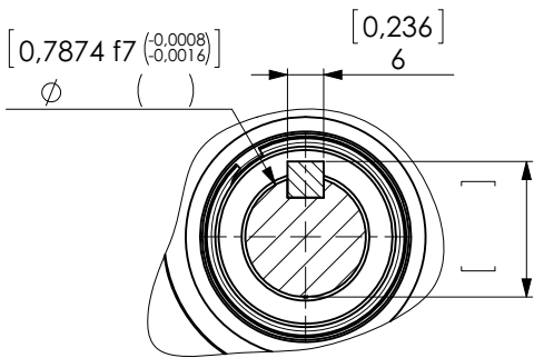
COUPE A-A
