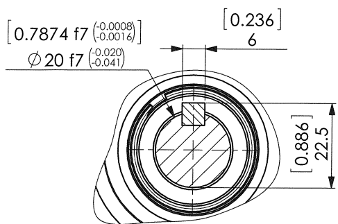
SEZIONE A-A
