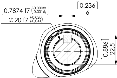
SEZIONE A-A
