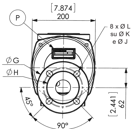
SEZIONE A-A
