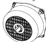
Deckel und Wellenpasselement, antriebsseitig
