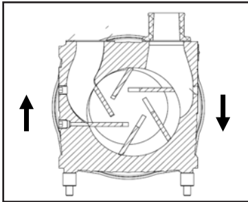
Abb. 3 - Drehrichtung
