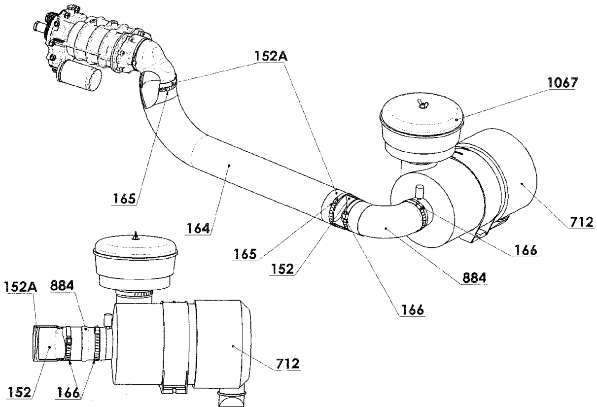
Luftfilter
