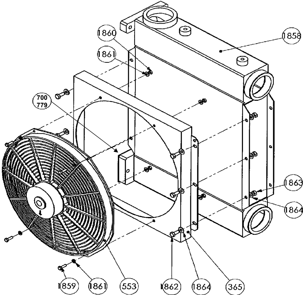
Lüftkuhler
