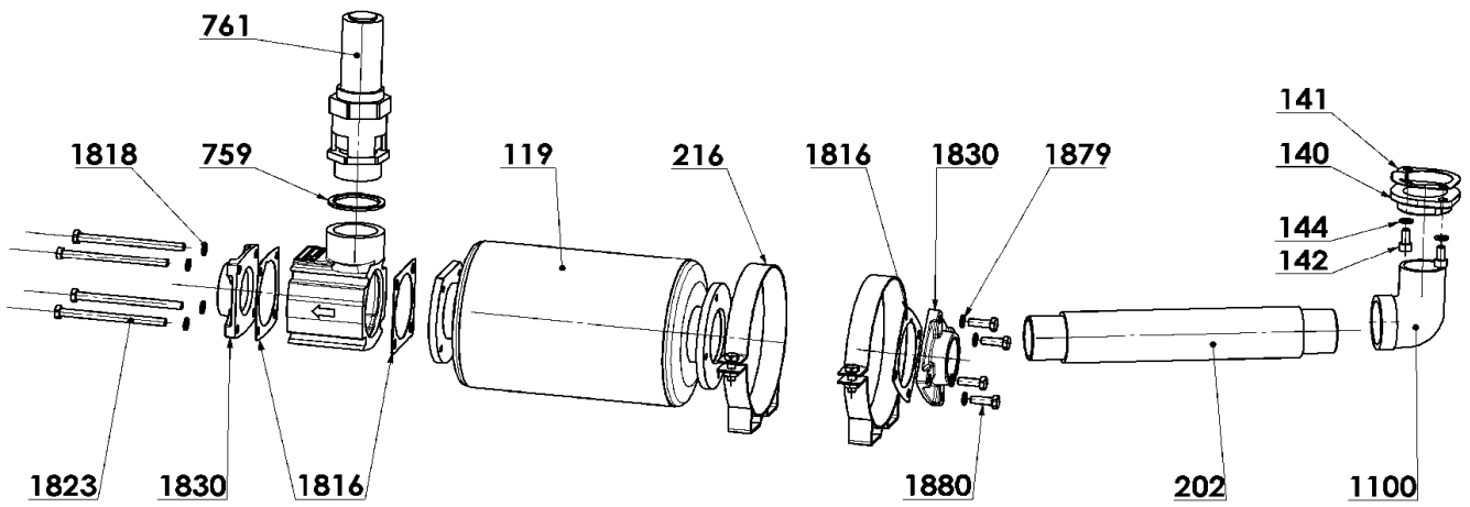
Schalldämpfer
